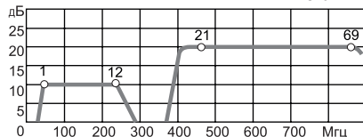
Типовая АЧХ
